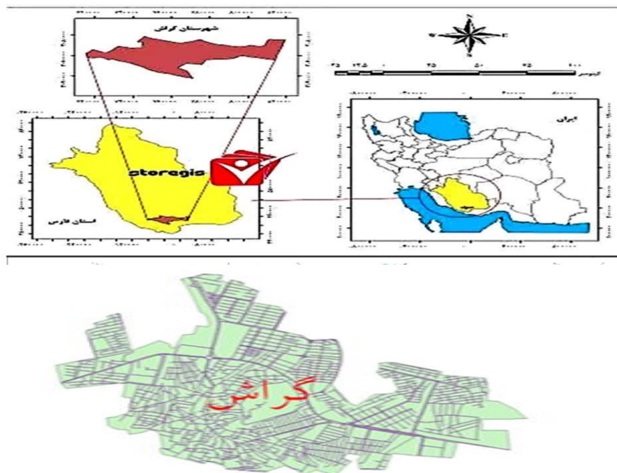
نقشه شماره یک- منطقه مورد مطالعه
