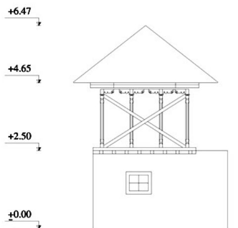
پلان شماری یک- طرح پلان و مقطع سفانفار اوکستر کریم کُلا (نگارندگان، ۱۳۸۸)
