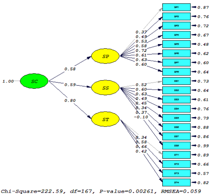
شکل شماره‌ی یک- مدل اندازه‌گیری سازه‌ی سرمایه‌ی اجتماعی در حالت تخمین استاندارد
